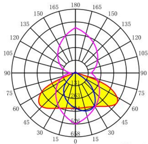
配光曲线
