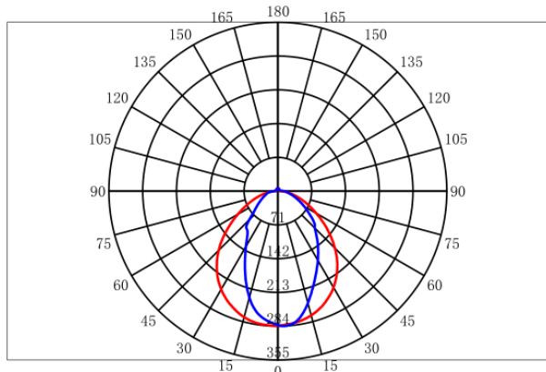
配光曲线
