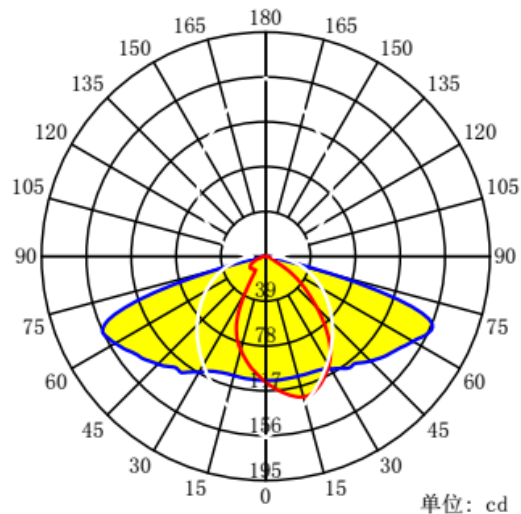
配光曲线
