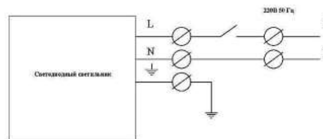
Рисунок 1. Схема подключения
