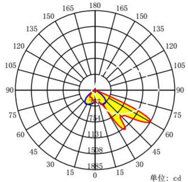
配光曲线
