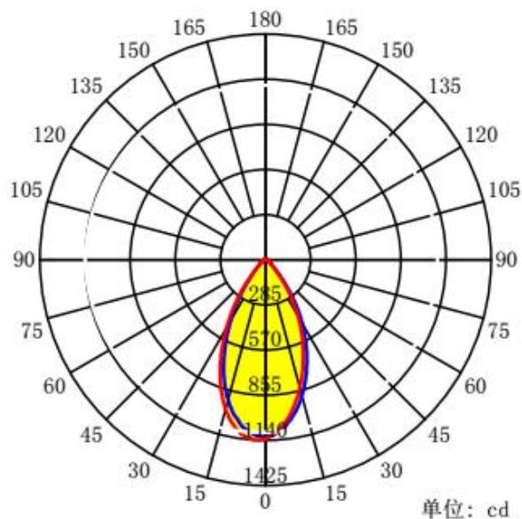
配光曲线
